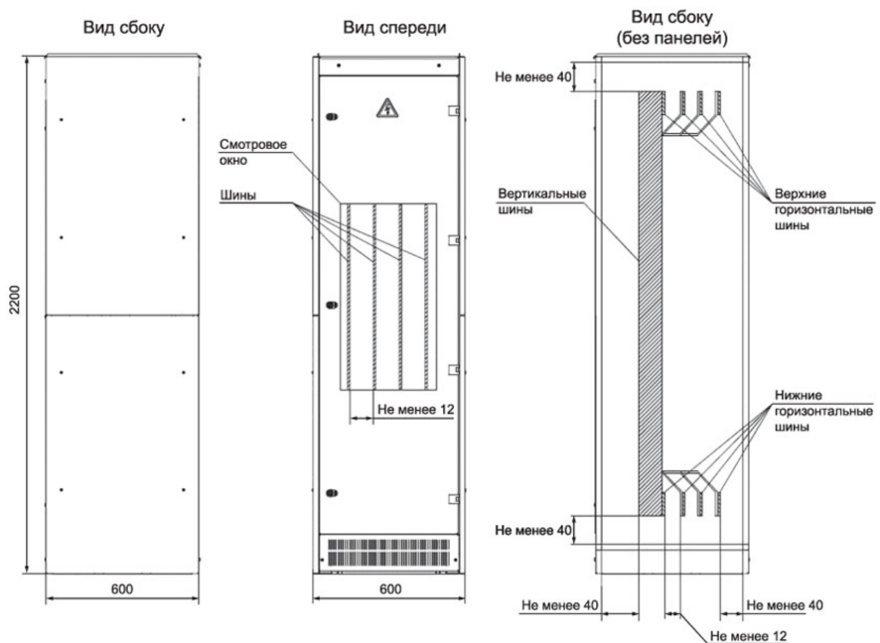
Рисунок Д.1 - Внешний вид металлического шкафа и размещение неизолированных токоведущих частей (шин)
