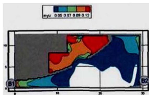
Рис. 77. Оптическая плотность дыма (Нп/м) в горизонтальном сечении на высоте 1,7 м от уровня пола в момент времени 200 с
