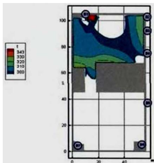
Рис. 29. Поля температуры (К) в горизонтальном сечении на высоте 1,7 м от уровня пола в момент времени 100 с
