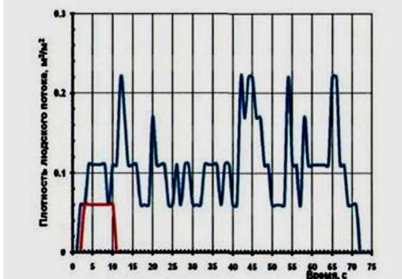
Рис. 124. Плотность людского потока на путях эвакуации (вариант 7):
