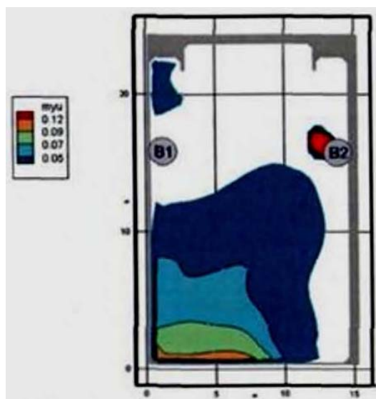
Рис. 86. Оптическая плотность дыма ( \text{Hп/м} ) в горизонтальном сечении на высоте 2,9 м от уровня пола в момент времени 170 с
