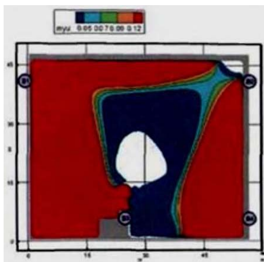
Рис. 15. Оптическая плотность дыма (Нп/м) в горизонтальном сечении на высоте 1,7 м от уровня пола в момент времени 100 с
