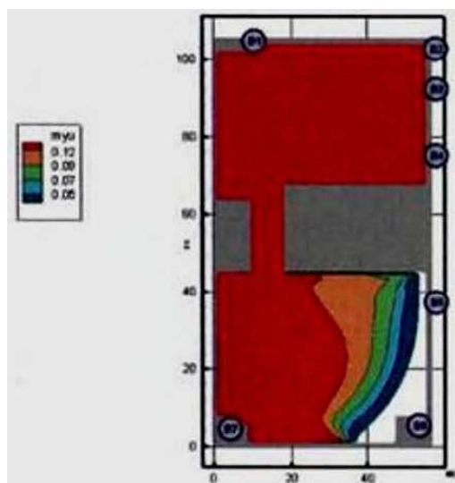
Рис 28. Оптическая плотность (Нп/м) в горизонтальном сечении на высоте 1,7 м от уровня пола в момент времени 300 с
