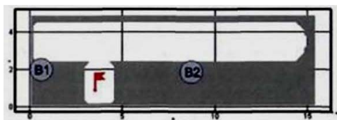
Рис. 128. Расчетная схема четвертого сценария развития пожара (горизонтальное сечение на высоте 1,7 м от уровня пола): В1, В2 - эвакуационные выходы
