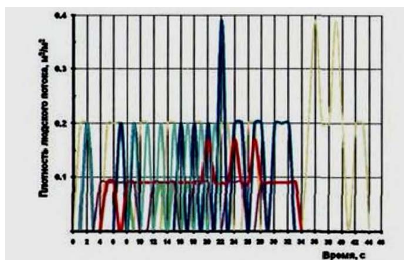
Рис. 117. Плотность людского потока на путях эвакуации (вариант 2):
