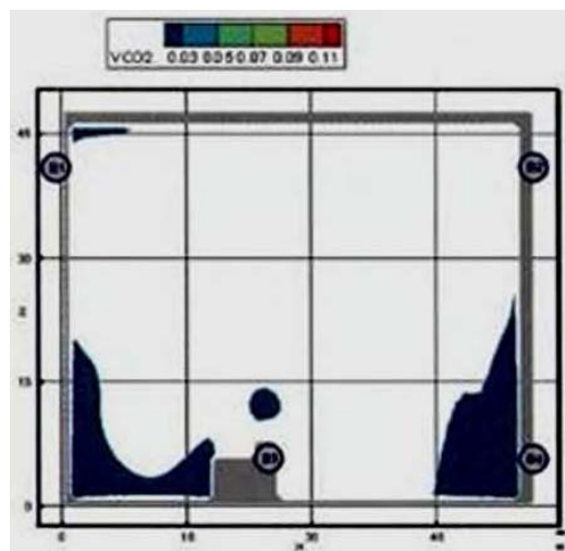
Рис. 18. Концентрация CO₂ (кг/м³) в горизонтальном сечении на высоте 1,7 м от уровня пола в момент времени 100 с
