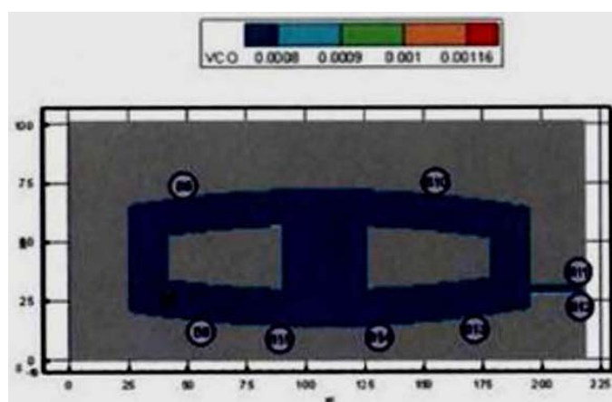
Рис. 64. Концентрация СО (кг/м³) в горизонтальном сечении на высоте 1,7 м от уровня пола второго этажа в момент времени 1100 с
