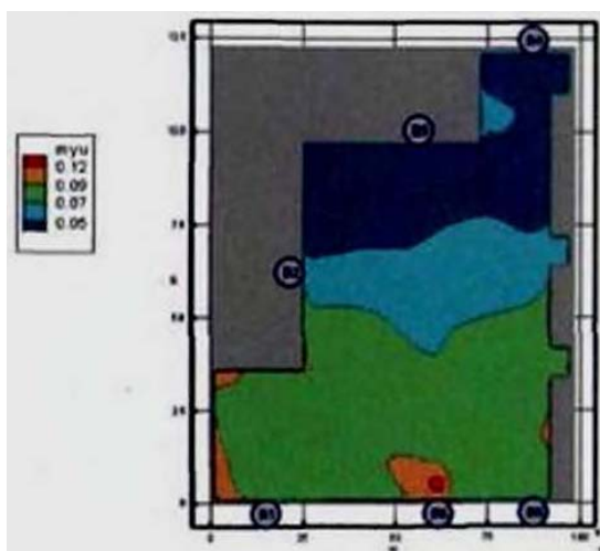
Рис. 42. Оптическая плотность дыма ( N_p/m ) в горизонтальном сечении на высоте 1,7 м от уровня пола в момент времени 1100 с
