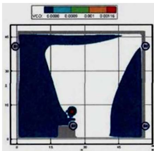
Рис. 17. Концентрация CO (кг/м³) в горизонтальном сечении на высоте 1,7 м от уровня пола в момент времени 100 с
