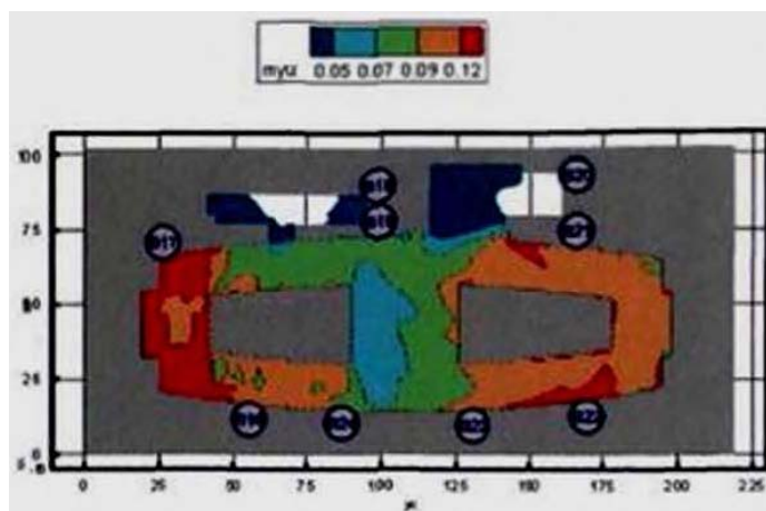
Рис. 54. Оптическая плотность дыма (Нп/м) в горизонтальном сечении на высоте 1,7 м от уровня пола третьего этажа в момент времени 840 с
