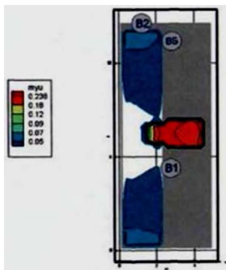
Рис. 154. Оптическая плотность дыма (Нп/м) в горизонтальном сечении на высоте 1,7 м от уровня пола в момент времени 100 с
