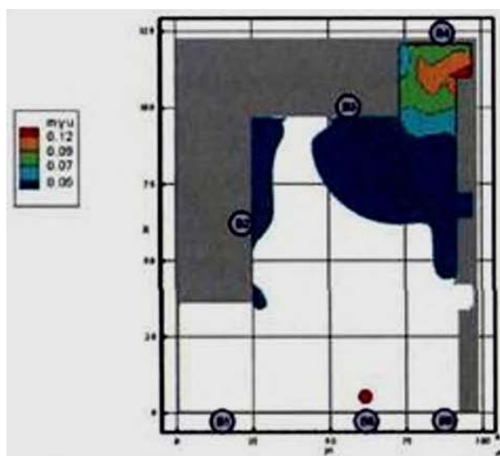
Рис. 40. Оптическая плотность дыма (Нп/м) в горизонтальном сечении на высоте 1,7 м от уровня пола в момент времени 700 с
