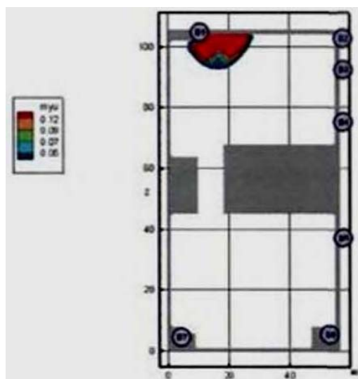
Рис. 22. Оптическая плотность дыма ( H_{п/м} ) в горизонтальном сечении на высоте 1,7 м от уровня пола в момент времени 20 с
