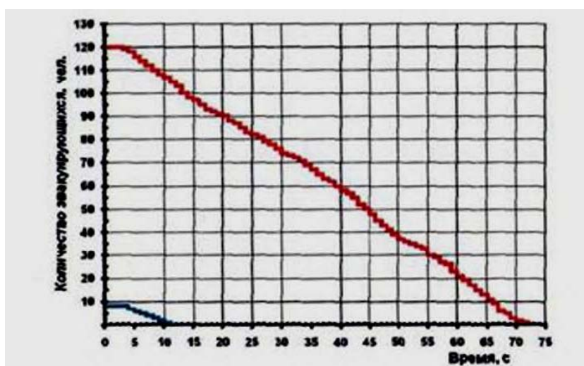
Рис. 115. Динамика эвакуации людей (вариант 7): — в выход В1; — в выход В2
