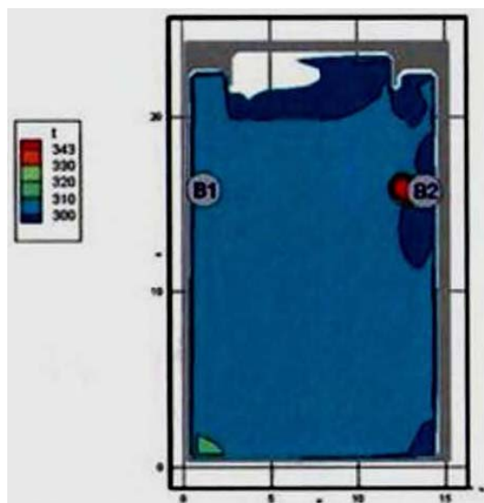
Рис. 90. Поля температуры (К) в горизонтальном сечении на высоте 2,9 м от уровня пола в момент времени 230 с
