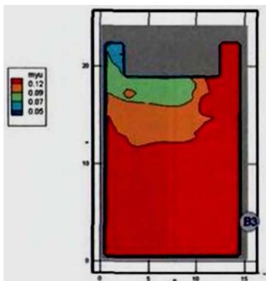
Рис. 88. Оптическая плотность дыма (Нп/м) в горизонтальном сечении на высоте 1,7 м от уровня пола в момент времени 410 с
