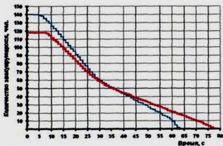
Рис. 114. Динамика эвакуации людей (вариант 6):
