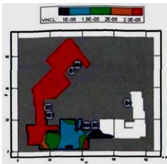
Рис. 151. Концентрация \text{HCl} ( \text{кг}/\text{м}^3 ) в горизонтальном сечении на высоте 1,7 м от уровня пола в момент времени 260 с
