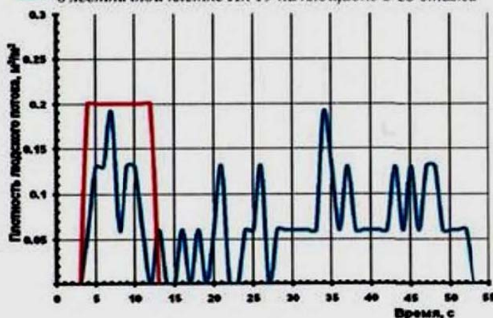
Рис. 122. Плотность людского потока на путях эвакуации (вариант 5):
