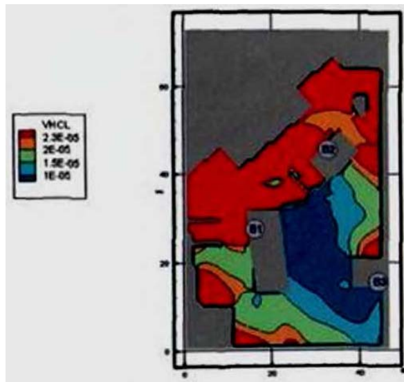
Рис. 138. Концентрация HCl ( \text{кг/м}^3 ) в горизонтальном сечении на высоте 1,7 м от уровня пола в момент времени 200 с
