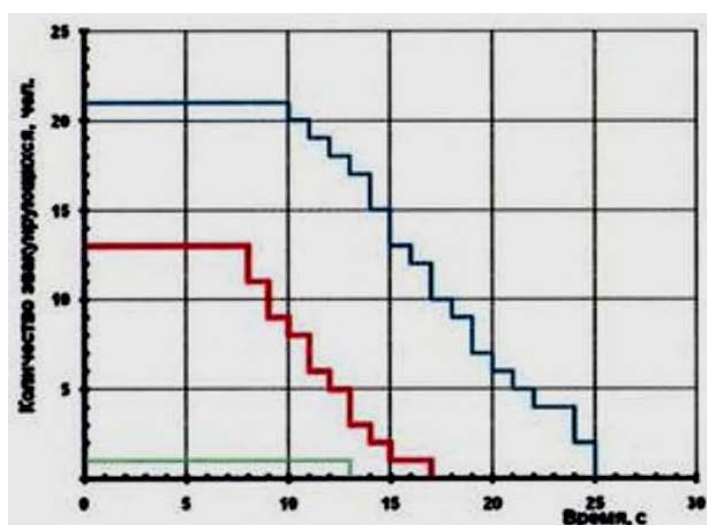
Рис. 171. Динамика эвакуации людей (вариант 2): — в выход В1; — в выход В3; — в выход В4
