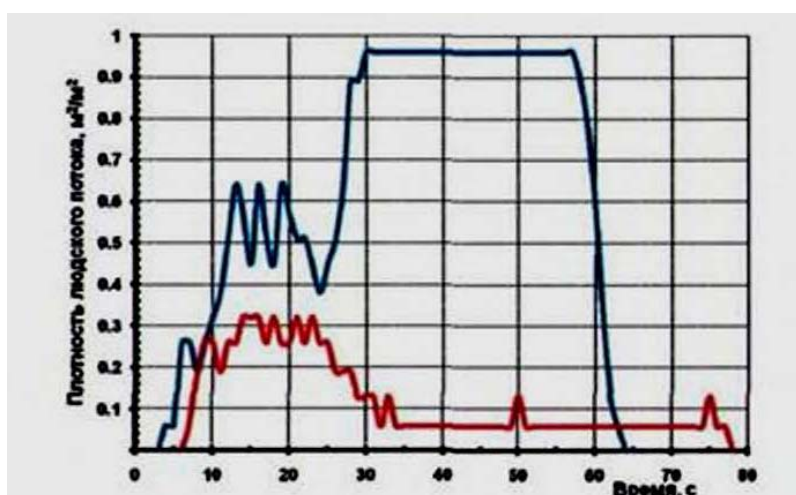
Рис. 123. Плотность людского потока на путях эвакуации (вариант 6):
