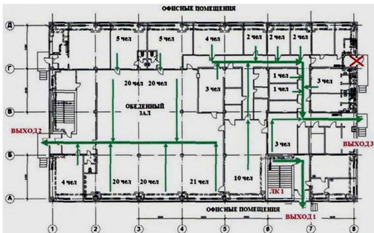
Рис. 190. Расчетная схема эвакуации с 1-го этажа
