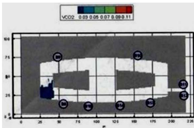
Рис. 67. Концентрация \text{CO}_2 ( \text{кг}/\text{м}^3 ) в горизонтальном сечении на высоте 1,7 м от уровня пола второго этажа в момент времени 1100 с
