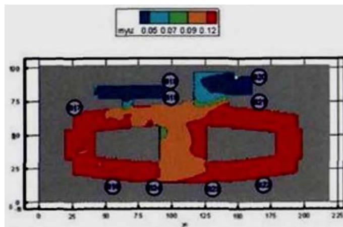
Рис. 57. Оптическая плотность дыма (Нп/м) в горизонтальном сечении на высоте 1,7 м от уровня пола третьего этажа в момент времени 940 с
