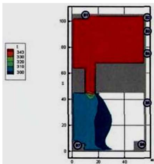
Рис. 30. Поля температуры (К) в горизонтальном сечении на высоте 1,7 м от уровня пола в момент времени 300 с
