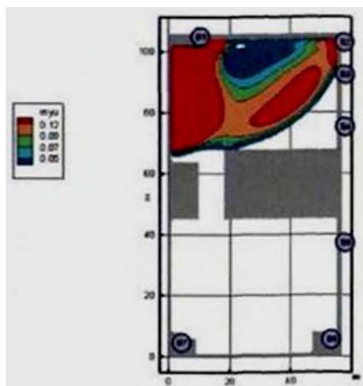
Рис. 24. Оптическая плотность дыма (Нп/м) в горизонтальном сечении на высоте 1,7 м от уровня пола в момент времени 70 с
