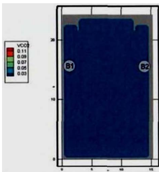
Рис. 94. Концентрация \text{CO}_2 ( \text{кг}/\text{м}^3 ) в горизонтальном сечении на высоте 2,9 м от уровня пола в момент времени 410 с
