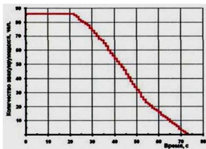
Рис. 174. Динамика эвакуации людей из здания наружу (вариант 4)
