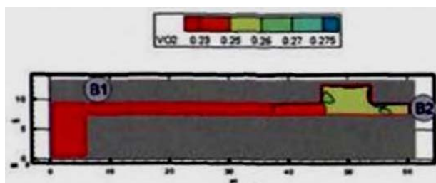
Рис. 108. Концентрация O_2 ( кг/м^3 ) в горизонтальном сечении на высоте 1,7 м от уровня пола в момент времени 290 с
