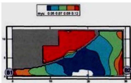
Рис. 78. Оптическая плотность дыма (Нп/м) в горизонтальном сечении на высоте 1,7 м от уровня пола в момент времени 220 с
