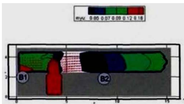
Рис. 162. Оптическая плотность дыма (Нп/м) в горизонтальном сечении на высоте 1,7 м от уровня пола в момент времени 150 с
