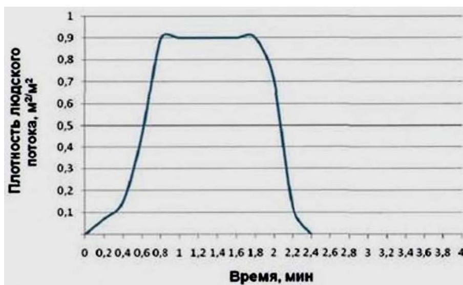
193. Зависимость плотности людского потока от времени на выходе с 3-го этажа в лестничную клетку
