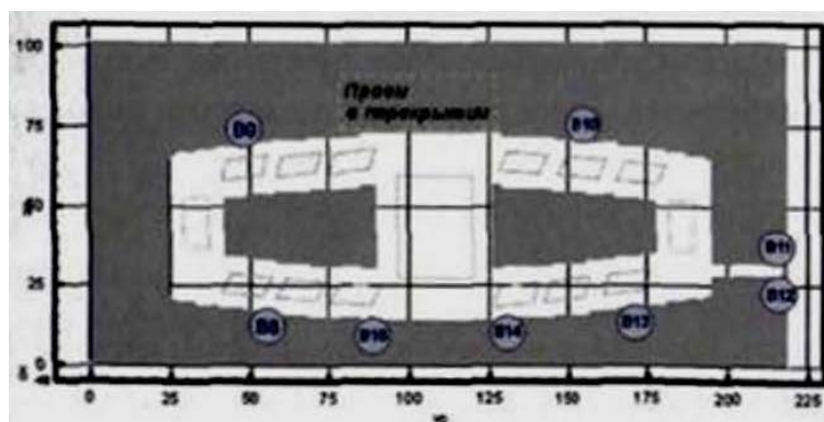
Рис. 5. Расчетная схема четвертого сценария развития пожара (горизонтальное сечение на высоте 1,7 м от уровня пола второго этажа): В8 - В15 - эвакуационные выходы
