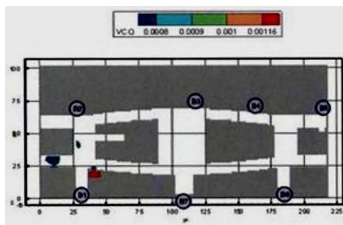
Рис. 63. Концентрация СО (кг/м 3 ) в горизонтальном сечении на высоте 1,7 м от уровня пола первого этажа в момент времени 1100 с
