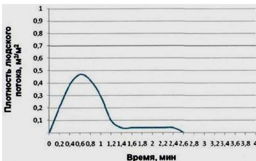
Рис. 196. Зависимость плотности людского потока от времени на лестничной площадке на уровне 2-го этажа
