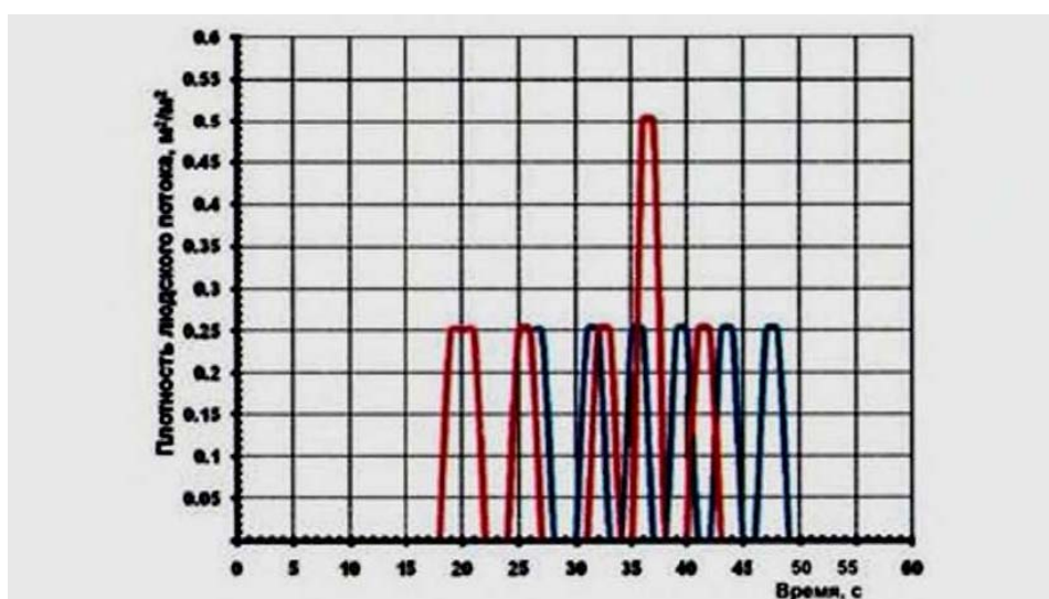
Рис. 177. Плотность людского потока на путях эвакуации (вариант 3):
