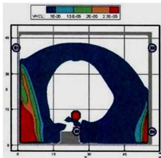
Рис 20. Концентрация HCl ( kg/m^3 ) в горизонтальном сечении на высоте 1,7 м от уровня пола в момент времени 70 с
