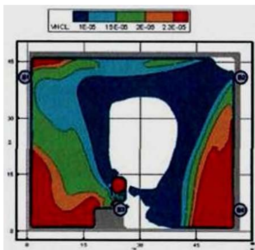
Рис. 21. Концентрация HCl ( \text{кг}/\text{м}^3 ) в горизонтальном сечении на высоте 1,7 м от уровня пола в момент времени 100 с
