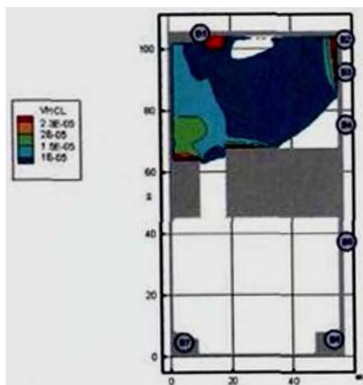
Рис. 36. Концентрация HCl (кг/м³) в горизонтальном сечении на высоте 1,7 м от уровня пола в момент времени 80 с
