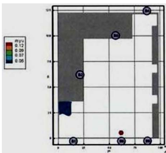
Рис. 39. Оптическая плотность дыма (Нп/м) в горизонтальном сечении на высоте 1,7 м от уровня пола в момент времени 400 с
