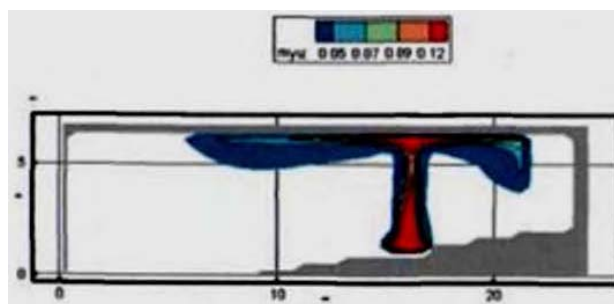
Рис. 84. Оптическая плотность дыма ( \text{Hп/м} ) в вертикальном сечении 1-1 в момент времени 80 с
