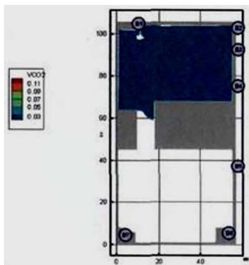
Рис. 32. Концентрация \text{CO}_2 ( \text{кг}/\text{м}^3 ) в горизонтальном сечении на высоте 1,7 м от уровня пола в момент времени 300 с
