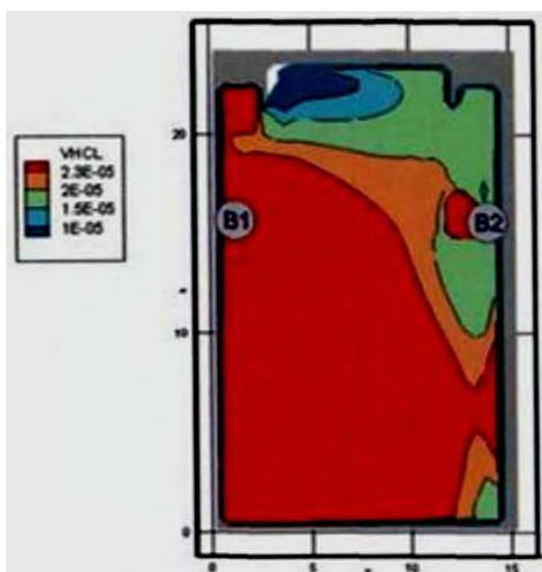
Рис. 98. Концентрация HCl (кг/м³) в горизонтальном сечении на высоте 1,7 м от уровня пола в момент времени 230 с
