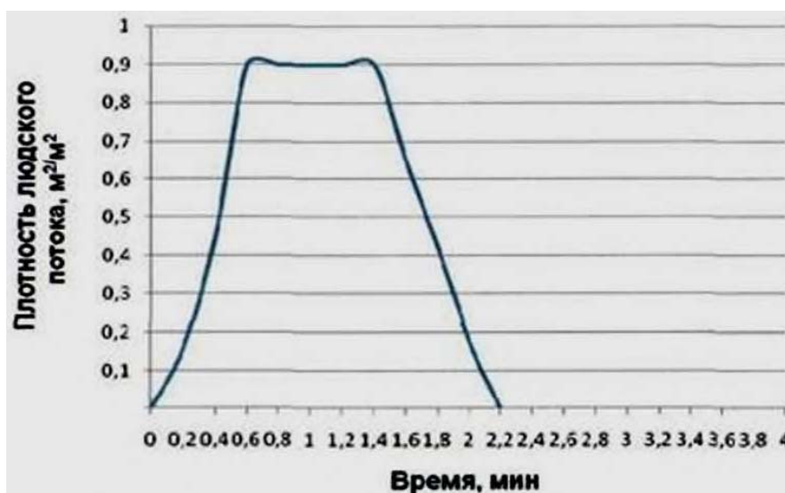
Рис. 198. Зависимость плотности людского потока от времени на выходе из здания (выход 2)
