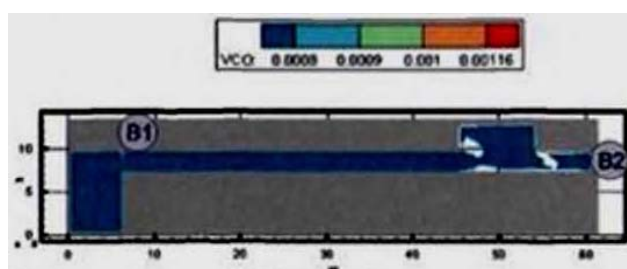
Рис. 105. Концентрация CO (кг/м³) в горизонтальном сечении на высоте 1,7 м от уровня пола в момент времени 290 с
