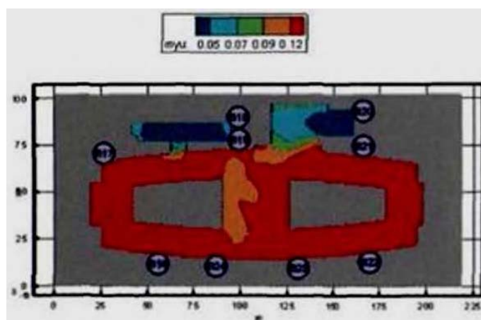
Рис. 58. Оптическая плотность дыма (Нп/м) в горизонтальном сечении на высоте 1,7 м от уровня пола третьего этажа в момент времени 980 с
