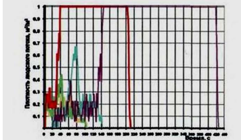
Рис. 118. Плотность людского потока на путях эвакуации (вариант 3):
