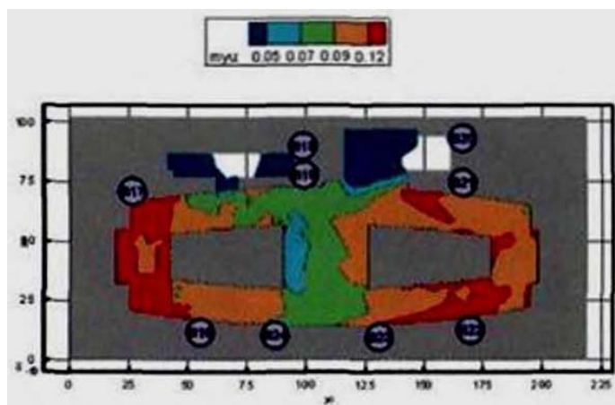
Рис. 55. Оптическая плотность дыма (Нп/м) в горизонтальном сечении на высоте 1,7 м от уровня пола третьего этажа в момент времени 860 с
