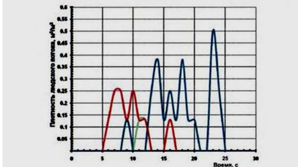
Рис. 176. Плотность людского потока на путях эвакуации (вариант 2):
