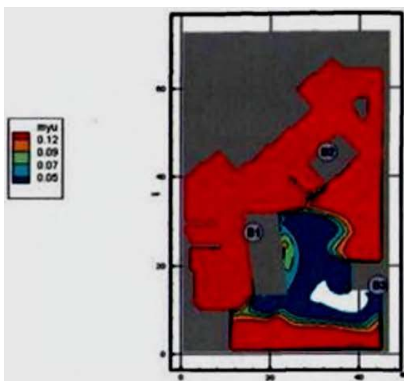
Рис. 132. Оптическая плотность дыма (Нп/м) в горизонтальном сечении на высоте 1,7 м от уровня пола в момент времени 170 с
