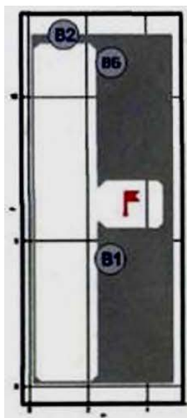
Рис. 127. Расчетная схема третьего сценария развития пожара (горизонтальное сечение на высоте 1,7 м от уровня пола): В1, В2 - эвакуационные выходы; ВБ вход в зону безопасности МГН
