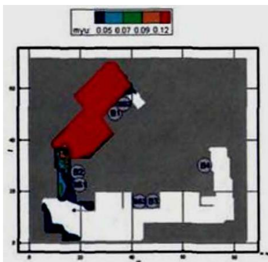
Рис. 141. Оптическая плотность дыма (Нп/м) в горизонтальном сечении на высоте 1,7 м от уровня пола в момент времени 120 с
