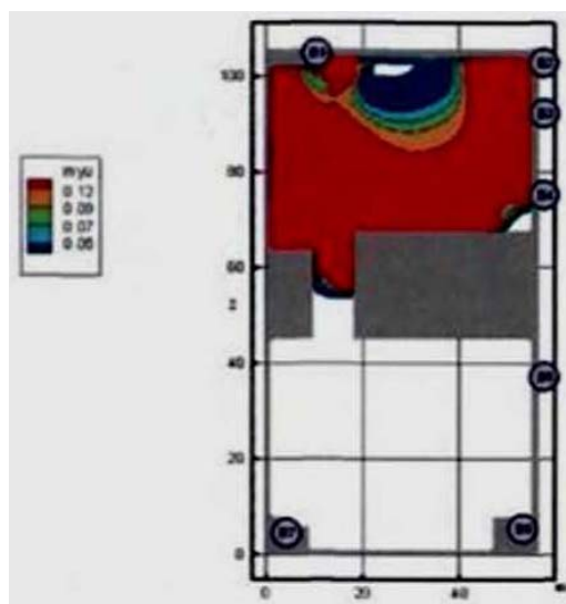
Рис. 26. Оптическая плотность дыма (Нп/м) в горизонтальном сечении на высоте 1,7 м от уровня пола в момент времени 100 с
