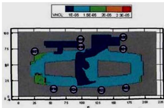
Рис. 72. Концентрация HCl ( кг/м^3 ) в горизонтальном сечении на высоте 1,7 м от уровня пола третьего этажа в момент времени 1100 с
