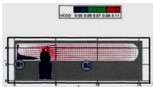
Рис. 167. Концентрация CO2 (кг/м³) в горизонтальном сечении на высоте 1,7 м от уровня пола в момент времени 190 с
