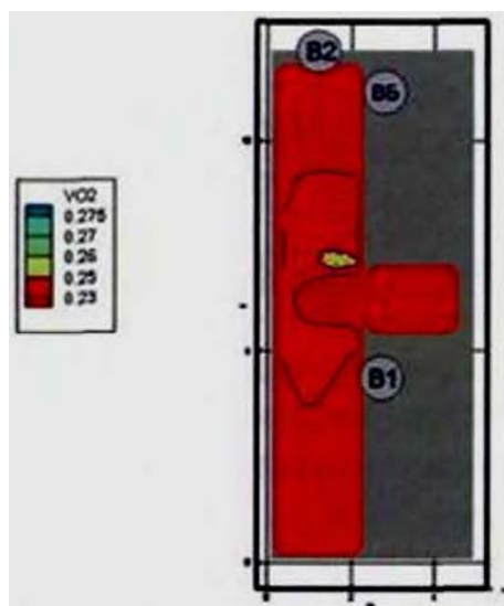
Рис. 186. Концентрация O_2 ( кг/м^3 ) в горизонтальном сечении на высоте 1,7 м от уровня пола в момент времени 180 с
