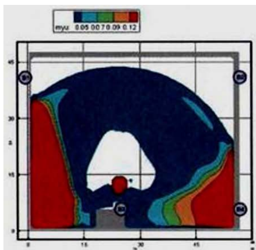
Рис. 13. Оптическая плотность дыма (Нп/м) в горизонтальном сечении на высоте 1,7 м от уровня пола в момент времени 70 с
