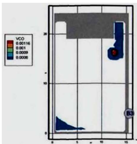
Рис 92. Концентрация СО (кг/м 3 ) в горизонтальном сечении на высоте 1,7 м от уровня пола в момент времени 410 с
