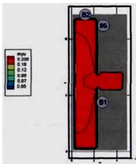
Рис. 155. Оптическая плотность дыма (Нп/м) в горизонтальном сечении на высоте 1,7 м от уровня пола в момент времени 160 с
