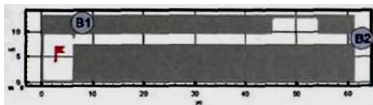
Рис. 10. Расчетная схема седьмого сценария развития пожара (горизонтальное сечение на высоте 1,7 м от уровня пола): B1, B2 - эвакуационные выходы
