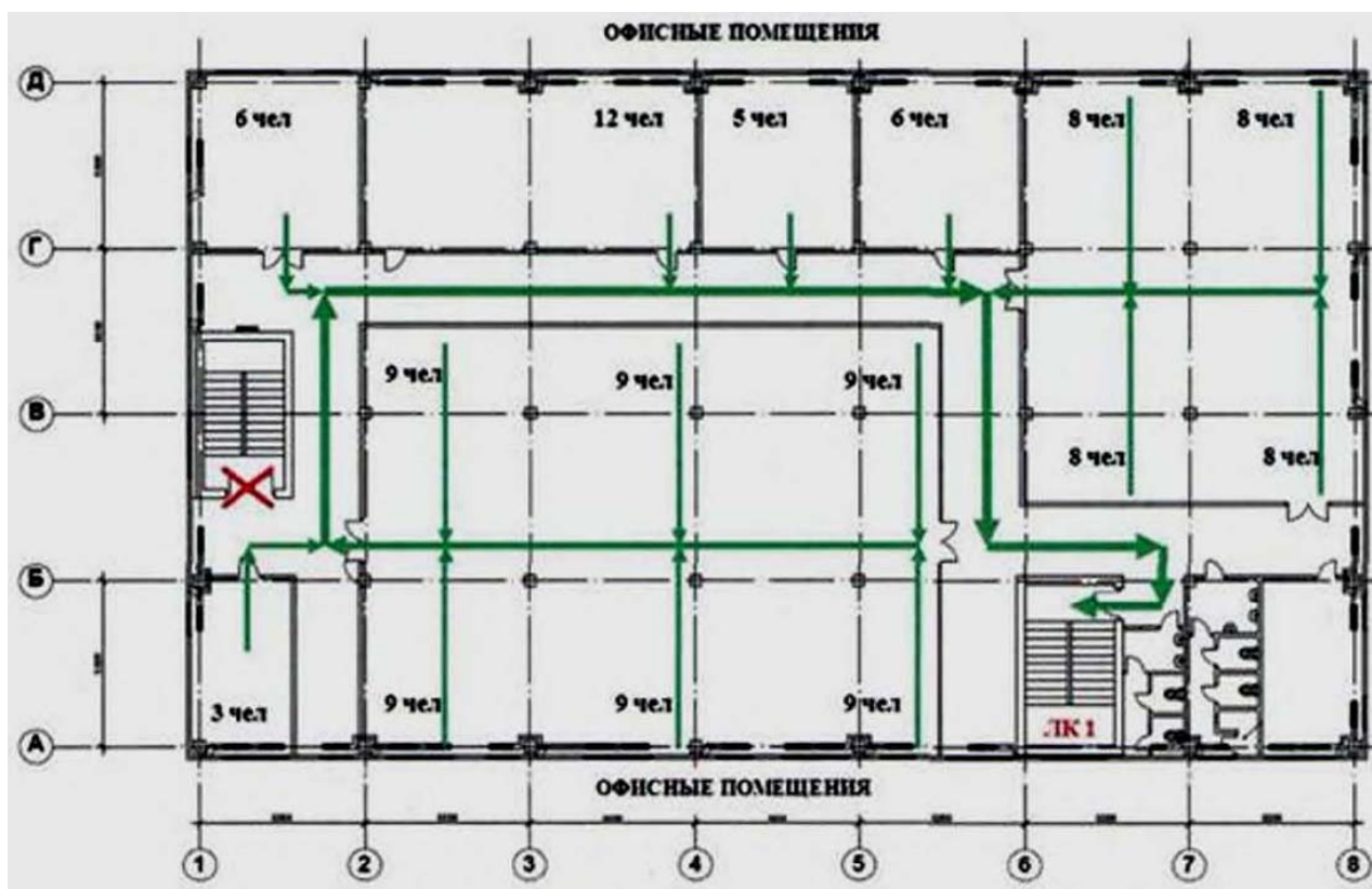
Рис. 192. Расчетная схема эвакуации с 3-го этажа
