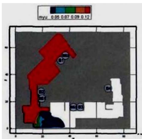
Рис. 142. Оптическая плотность дыма (Нп/м) в горизонтальном сечении на высоте 1,7 м от уровня пола в момент времени 170 с
