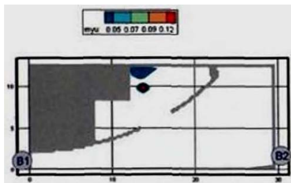
Рис. 75. Оптическая плотность дыма (Нп/м) в горизонтальном сечении на высоте 1,7 м от уровня пола в момент времени 60 с
