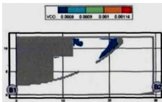
Рис. 80. Концентрация CO (кг/м³) в горизонтальном сечении на высоте 1,7 м от уровня пола в момент времени 220 с
