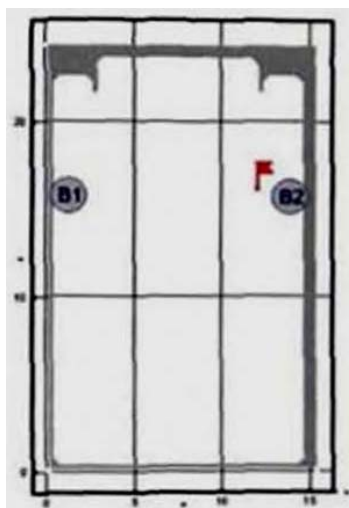
Рис. 9. Расчетная схема шестого сценария развития пожара (горизонтальное сечение на высоте 2,9 м от уровня пола): B1, B2 - эвакуационные выходы
