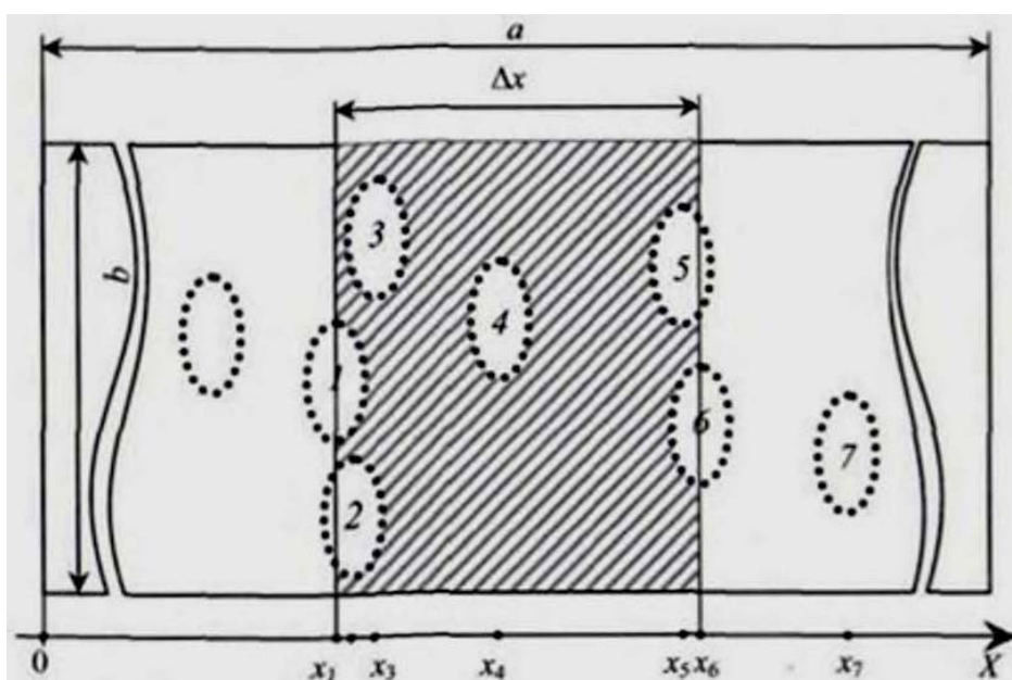
Рис. 109. Координатная схема размещения людей на путях эвакуации
