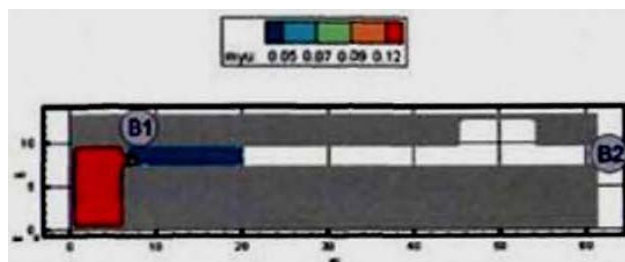
Рис. 100. Оптическая плотность дыма (Нп/м) в горизонтальном сечении на высоте 1,7 м от уровня пола в момент времени 150 с
