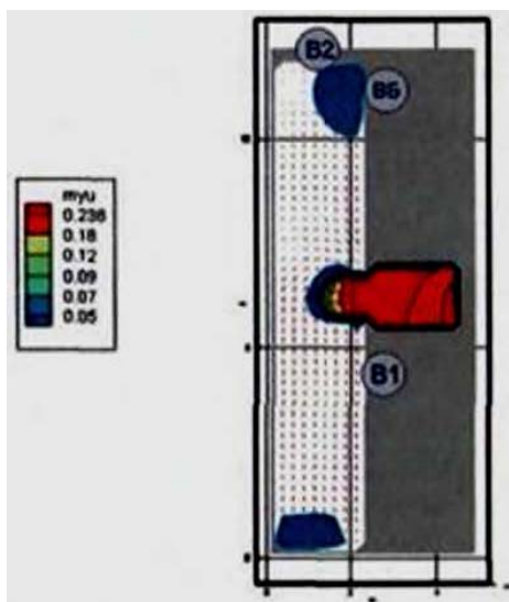
Рис. 180. Оптическая плотность дыма (Нп/м) в горизонтальном сечении на высоте 1,7 м от уровня пола в момент времени 100 с
