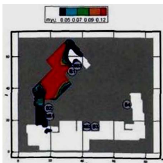
Рис. 140. Оптическая плотность дыма (Нп/м) в горизонтальном сечении на высоте 1,7 м от уровня пола в момент времени 100 с
