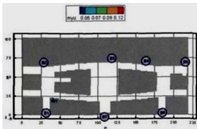
Рис. 48. Оптическая плотность дыма (Нп/м) в горизонтальном сечении на высоте 1,7 м от уровня пола первого этажа в момент времени 80 с
