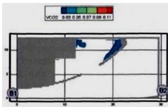
Рис. 81. Концентрация CO 2 (кг/м 3 ) в горизонтальном сечении на высоте 1,7 м от уровня пола в момент времени 220 с
