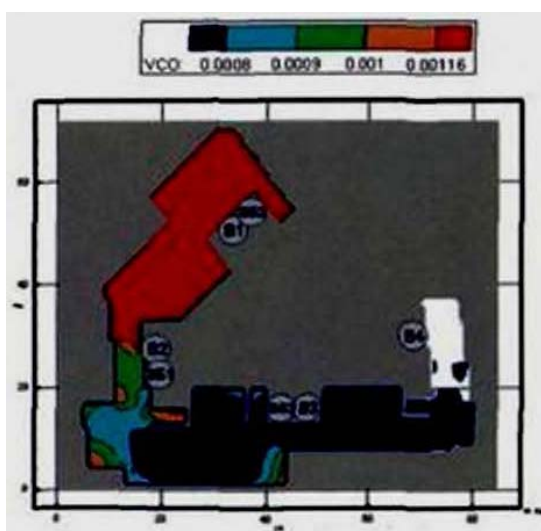
Рис. 148. Концентрация CO (кг/м³) в горизонтальном сечении на высоте 1,7 м от уровня пола в момент времени 430 с
