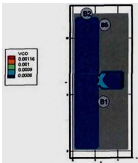
Рис. 157. Концентрация CO (кг/м³) в горизонтальном сечении на высоте 1,7 м от уровня пола в момент времени 160 с
