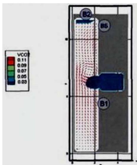
Рис. 185. Концентрация CO 2 (кг/м³) в горизонтальном сечении на высоте 1,7 м от уровня пола в момент времени 180 с
