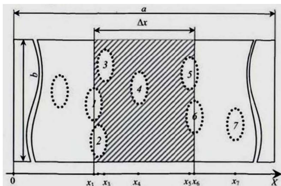
Рис. 169. Координатная схема размещения людей на путях эвакуации
