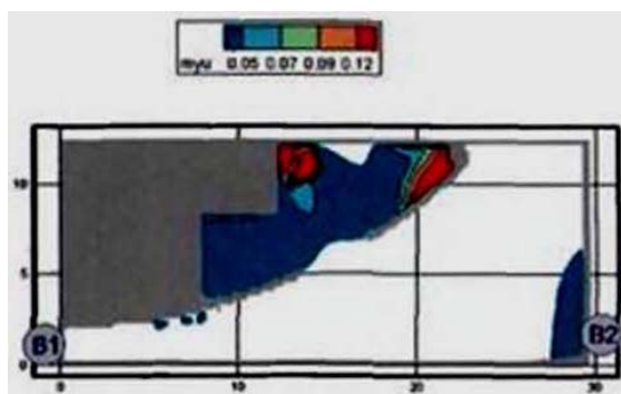
Рис. 76. Оптическая плотность дыма (Нп/м) в горизонтальном сечении на высоте 1,7 м от уровня пола в момент времени 150 с
