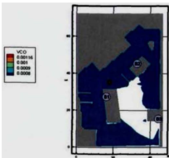
Рис. 135. Концентрация СО (кг/м³) в горизонтальном сечении на высоте 1,7 м от уровня пола в момент времени 200 с
