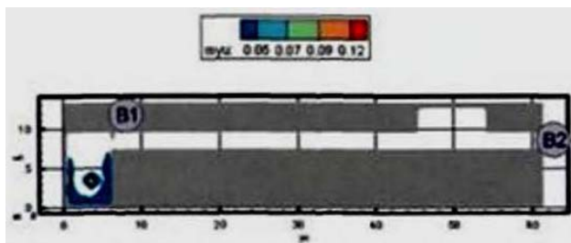
Рис. 99. Оптическая плотность дыма ( Hп/м ) в горизонтальном сечении на высоте 1,7 м от уровня пола в момент времени
