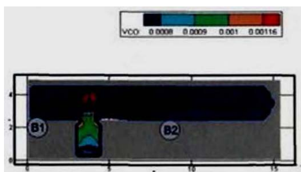
Рис. 166. Концентрация CO (кг/м³) в горизонтальном сечении на высоте 1,7 м от уровня пола в момент времени 190 с
