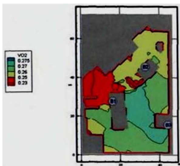
Рис. 137. Концентрация \text{O}_2 ( \text{кг}/\text{м}^3 ) в горизонтальном сечении на высоте 1,7 м от уровня пола в момент времени 200 с
