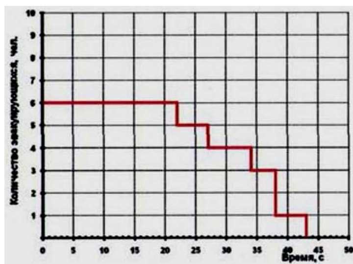
Рис. 172. Динамика эвакуации людей с этажа (вариант 3)
