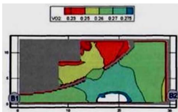
Рис. 82. Концентрация O 2 (кг/м 3 ) в горизонтальном сечении на высоте 1,7 м от уровня пола в момент времени 220 с
