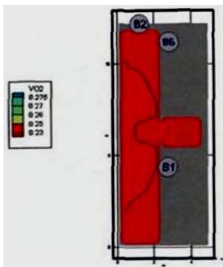
Рис. 159. Концентрация O_2 ( кг/м^3 ) в горизонтальном сечении на высоте 1,7 м от уровня пола в момент времени 160 с
