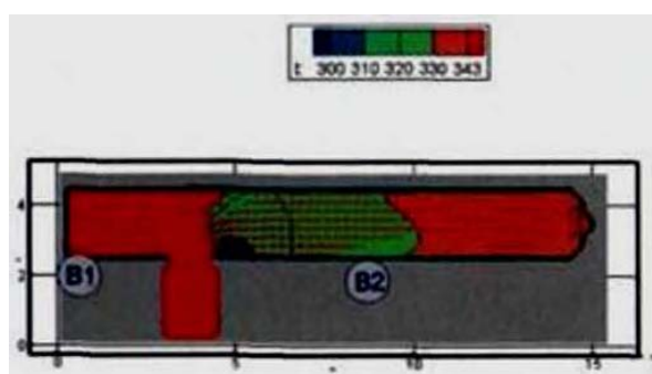
Рис 165. Поля температуры (К) в горизонтальном сечении на высоте 1,7 м от уровня пола в момент времени 190 с
