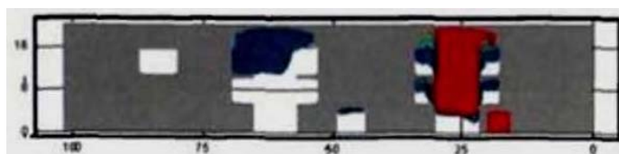
Рис 50. Оптическая плотность дыма (Нп/м) в вертикальном сечении 1-1 в момент времени 400 с
