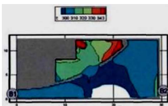
Рис. 79. Поля температуры (K) в горизонтальном сечении на высоте 1,7 м от уровня пола в момент времени 220 с
