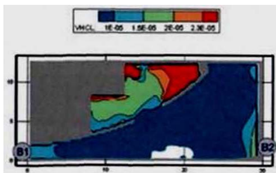
Рис. 83. Концентрация HCl (кг/м 3 ) в горизонтальном сечении на высоте 1,7 м от уровня пола в момент времени 220 с
