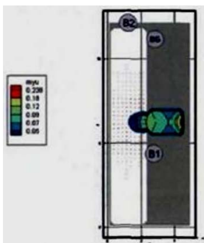
Рис. 179. Оптическая плотность дыма (Нп/м) в горизонтальном сечении на высоте 1,7 м от уровня пола в момент времени 60 с
