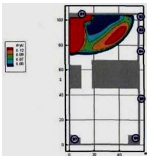
Рис. 23. Оптическая плотность дыма ( H_{п/м} ) в горизонтальном сечении на высоте 1,7 м от уровня пола в момент времени 60 с
