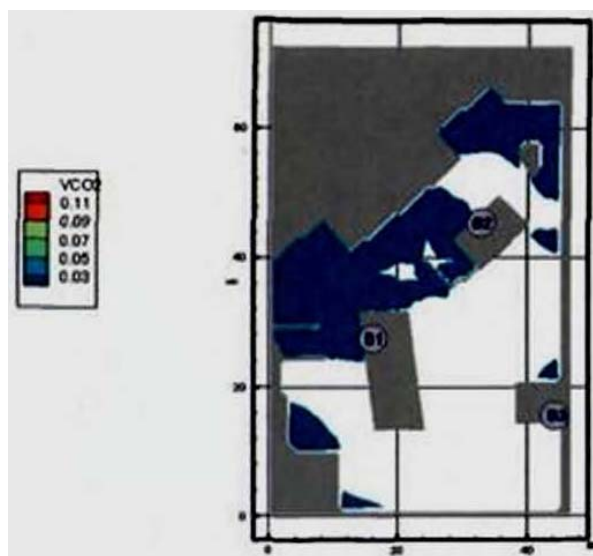
Рис. 136. Концентрация \text{CO}_2 ( \text{кг}/\text{м}^3 ) в горизонтальном сечении на высоте 1,7 м от уровня пола в момент времени 200 с
