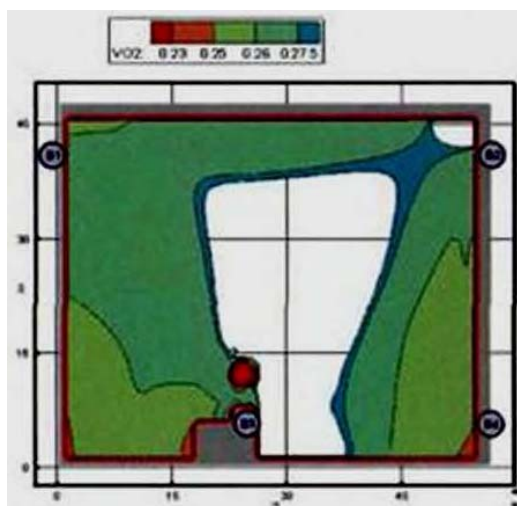
Рис. 19. Концентрация O_2 ( kg/m^3 ) в горизонтальном сечении на высоте 1,7 м от уровня пола в момент времени 100 с
