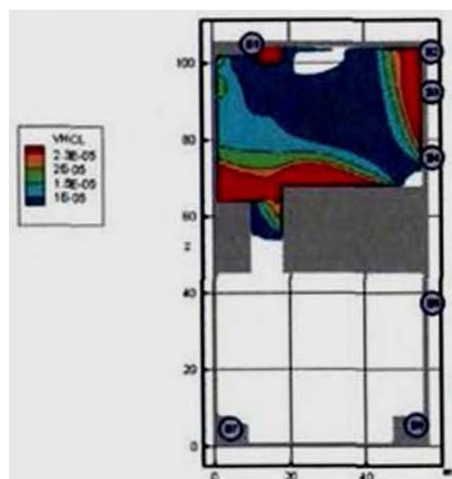
Рис. 37. Концентрации HCl (кг/м³) в горизонтальном сечении на высоте 1,7 м от уровня пола в момент времени 100 с
