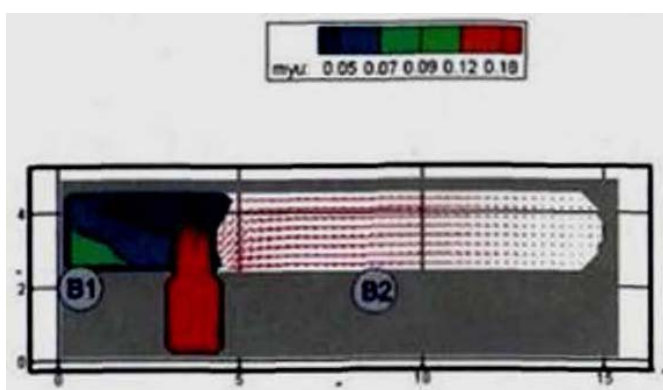
Рис. 161. Оптическая плотность дыма (Нп/м) в горизонтальном сечении на высоте 1,7 м от уровня пола в момент времени 110 с
