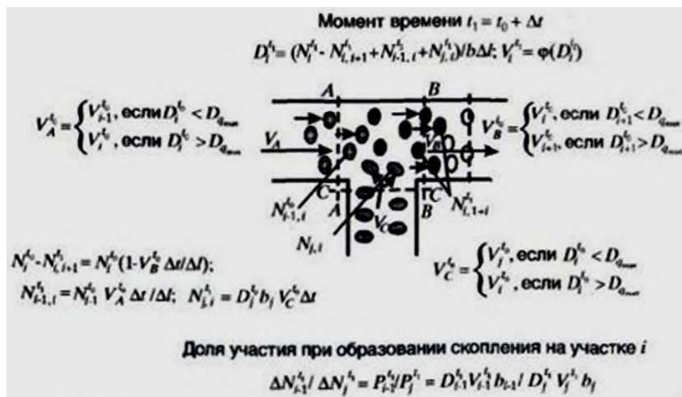
Рис. 189. Изменения состояния потока в последовательные моменты времени
