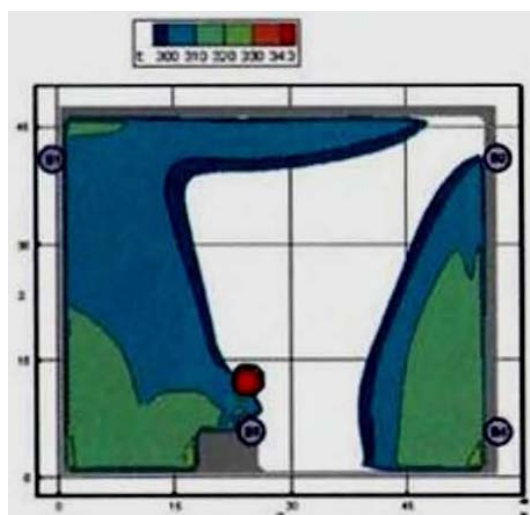
Рис. 16. Поля температуры (К) в горизонтальном сечении на высоте 1,7 м от уровня пола в момент времени 100 с
