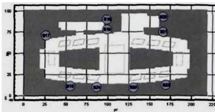
Рис. 6. Расчетная схема четвертого сценария развития пожара (горизонтальное сечение на высоте 1,7 м от уровня пола третьего этажа): В16 - В24 эвакуационные выходы
