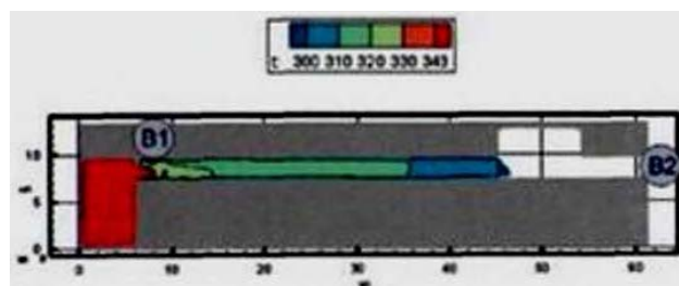
Рис. 103. Поля температуры (К) в горизонтальном сечении
