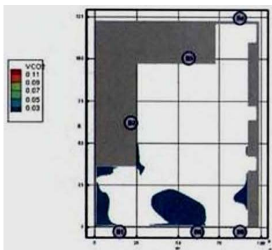
Рис. 45. Концентрация CO₂ (кг/м³) в горизонтальном сечении на высоте 1,7 м от уровня пола в момент времени 1100 с
