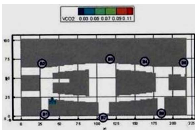
Рис. 68. Концентрация \text{CO}_2 ( \text{кг}/\text{м}^3 ) в горизонтальном сечении на высоте 1,7 м от уровня пола первого этажа в момент времени 1100 с
