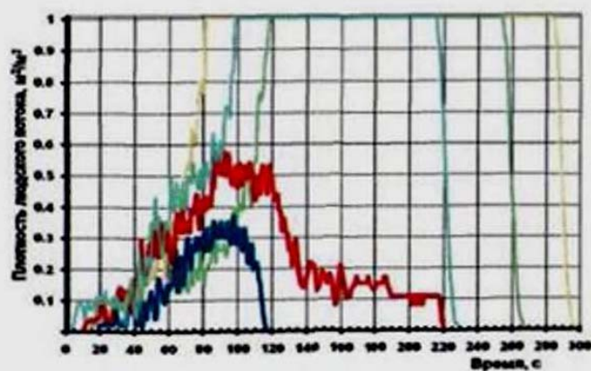
Рис. 120. Плотность людского потока на путях эвакуации (вариант 4):
