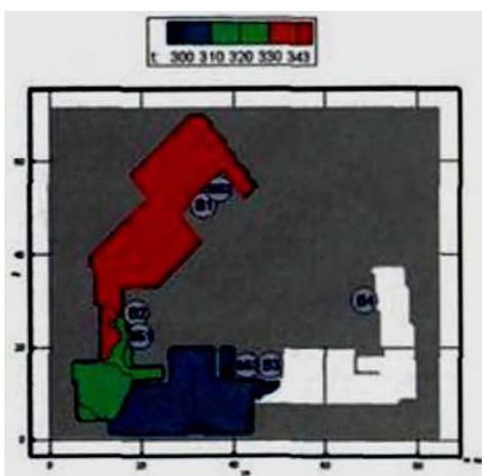
Рис. 146. Поля температуры (К) в горизонтальном сечении на высоте 1,7 м от уровня пола в момент времени 260 с
