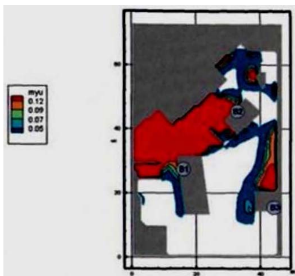
Рис. 130. Оптическая плотность дыма (Нп/м) в горизонтальном сечении на высоте 1,7 м от уровня пола в момент времени 110 с
