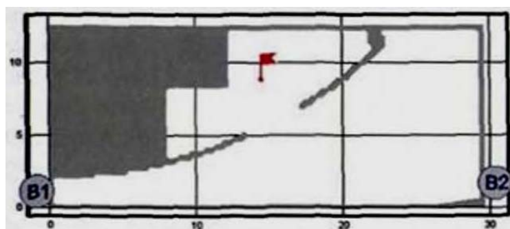
Рис. 7. Расчетная схема пятого сценария развития пожара (горизонтальное сечение на высоте 1,7 м от уровня пола): B1, B2 - эвакуационные выходы
