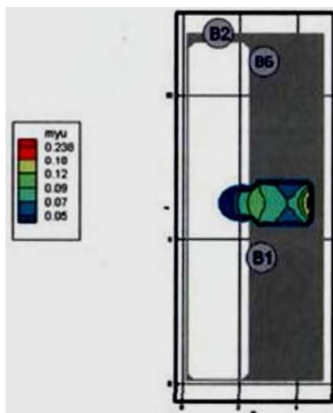
Рис. 153. Оптическая плотность дыма (Нп/м) в горизонтальном сечении на высоте 1,7 м от уровня пола в момент времени 60 с
