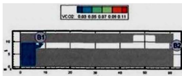
Рис. 106. Концентрация CO2 (кг/м³) в горизонтальном сечении на высоте 1,7 м от уровня пола в момент времени 290 с
