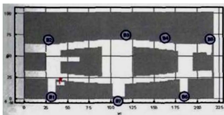
Рис. 4. Расчетная схема четвертого сценария развития пожара (горизонтальное сечение на высоте 1,7 м от уровня пола первого этажа): В1 - В7 эвакуационные выходы
