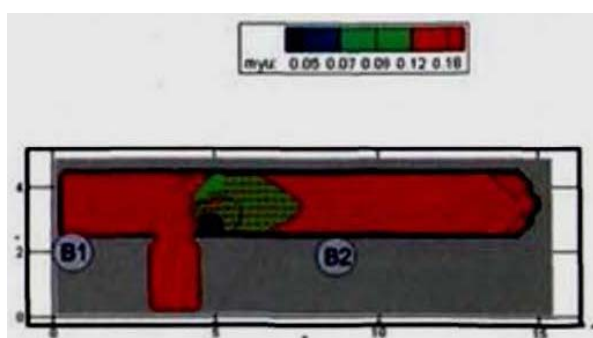
Рис. 163. Оптическая плотность дыма (Нп/м) в горизонтальном сечении на высоте 1,7 м от уровня пола в момент времени 170 с
