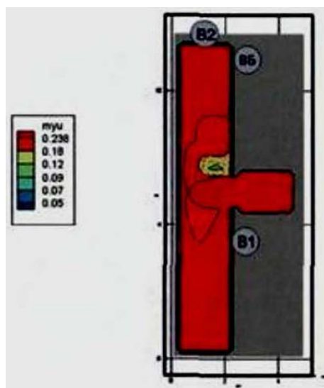
Рис. 182. Оптическая плотность дыма ( H_{п/м} ) в горизонтальном сечении на высоте 1,7 м от уровня пола в момент времени 180 с
