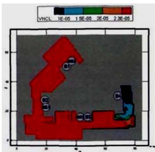
Рис. 152. Концентрация \text{HCl} ( \text{кг}/\text{м}^3 ) в горизонтальном сечении на высоте 1,7 м от уровня пола в момент времени 430 с
