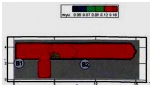
Рис. 164. Оптическая плотность дыма (Нп/м) в горизонтальном сечении на высоте 1,7 м от уровня пола в момент времени 190 с
