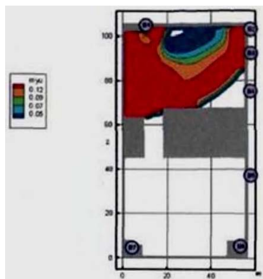
Рис 25. Оптическая плотность дыма (Нп/м) в горизонтальном сечении на высоте 1,7 м от уровня пола в момент времени 80 с
