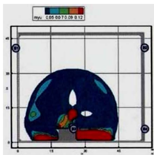
Рис. 12. Оптическая плотность дыма (Нп/м) в горизонтальном сечении на высоте 1,7 м от уровня пола в момент времени 40 с
