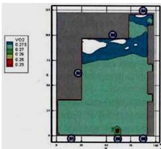
Рис. 46. Концентрация O_2 ( кг/м^3 ) в горизонтальном сечении на высоте 1,7 м от уровня пола в момент времени 1100 с
