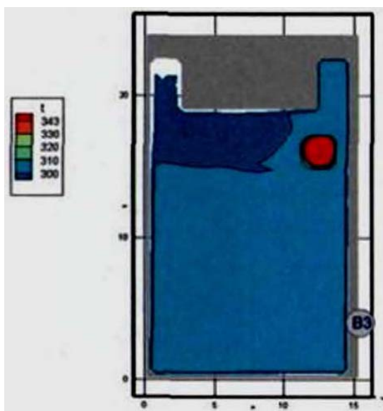
Рис. 89. Поля температуры (К) в горизонтальном сечении на высоте 1,7 м от уровня пола в момент времени 410 с
