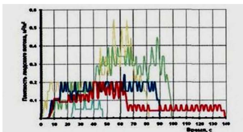
Рис. 121. Плотность людского потока на путях эвакуации (вариант 4):
