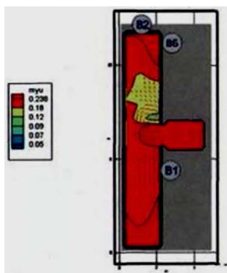
Рис. 181. Оптическая плотность дыма (Нп/м) в горизонтальном сечении на высоте 1,7 м от уровня пола в момент времени 170 с
