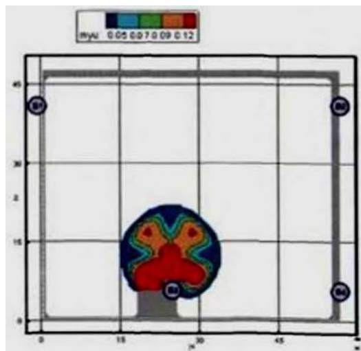
Рис. 11. Оптическая плотность дыма (Нп/м) в горизонтальном сечении на высоте 1,7 м от уровня пола в момент времени 20 с
