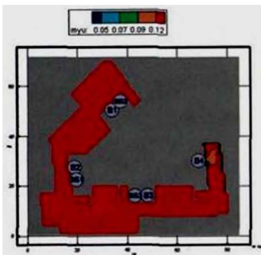
Рис. 145. Оптическая плотность дыма (Нп/м) в горизонтальном сечении на высоте 1,7 м от уровня пола в момент времени 430 с
