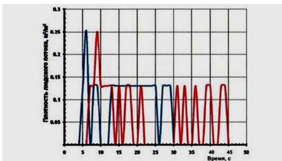
Рис. 175. Плотность людского потока на путях эвакуации (вариант 1):
