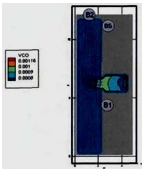
Рис. 184. Концентрация CO (кг/м³) в горизонтальном сечении на высоте 1,7 м от уровня пола в момент времени 180 с
