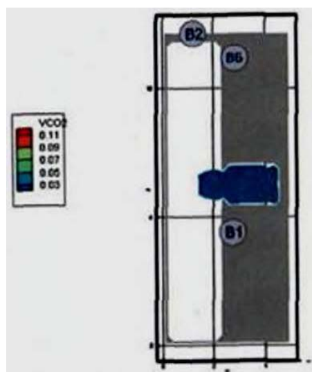
Рис. 158. Концентрация CO2 (кг/м³) в горизонтальном сечении на высоте 1,7 м от уровня пола в момент времени 160 с
