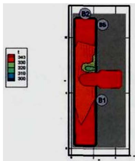
Рис. 183. Поля температуры ( K ) в горизонтальном сечении на высоте 1,7 м от уровня пола в момент времени 180 с
