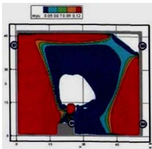
Рис. 14. Оптическая плотность дыма (Нп/м) в горизонтальном сечении на высоте 1,7 м от уровня пола в момент времени 90 с
