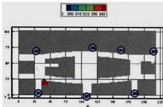
Рис. 62. Поля температуры (К) в горизонтальном сечении на высоте 1,7 м от уровня пола первого этажа в момент времени 1100 с
