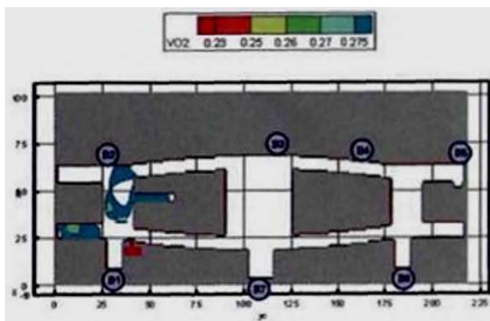
Рис. 69. Концентрация O_2 ( кг/м^3 ) в горизонтальном сечении на высоте 1,7 м от уровня пола первого этажа в момент времени 1100 с
