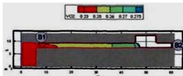
Рис. 107. Концентрация O2 (кг/м³) в горизонтальном сечении на высоте 1,7 м от уровня пола в момент времени 230 с
