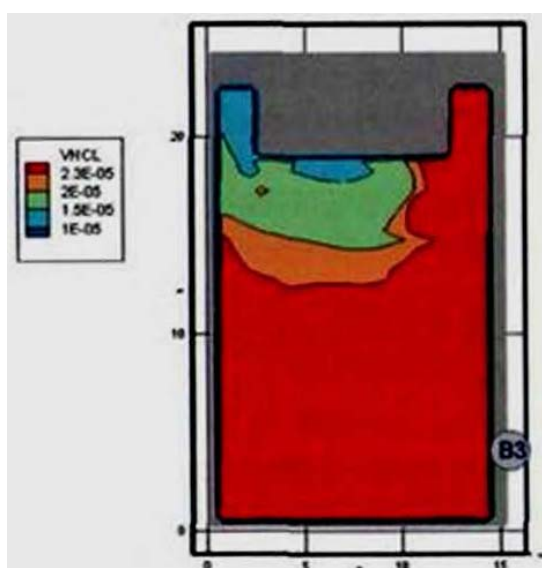
Рис. 97. Концентрация HCl (кг/м³) в горизонтальном сечении на высоте 1,7 м от уровня пола в момент времени 410 с
