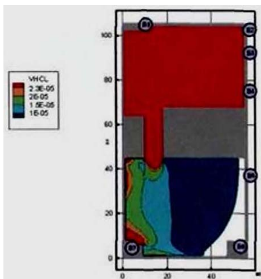
Рис. 38. Концентрации HCl ( \text{кг/м}^3 ) в горизонтальном сечении на высоте 1,7 м от уровня пола в момент времени 300 с
