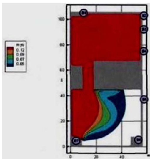
Рис. 27. Оптическая плотность дыма (Нп/м) в горизонтальном сечении на высоте 1,7 м от уровня пола в момент времени 250 с
