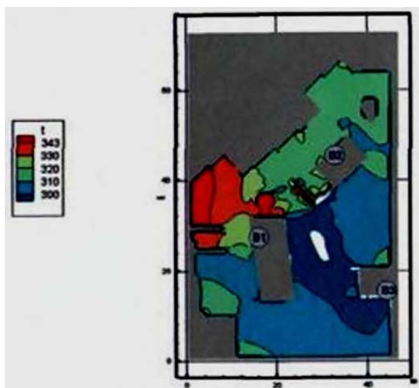
Рис. 134. Поля температуры (К) в горизонтальном сечении на высоте 1,7 м от уровня пола в момент времени 200 с
