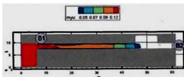
Рис. 101. Оптическая плотность дыма (Нп/м) в горизонтальном сечении на высоте 1,7 м от уровня пола в момент времени 230 с
