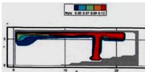
Рис. 85. Оптическая плотность дыма ( \text{Hп/м} ) в вертикальном сечении 1-1 в момент времени 130 с
