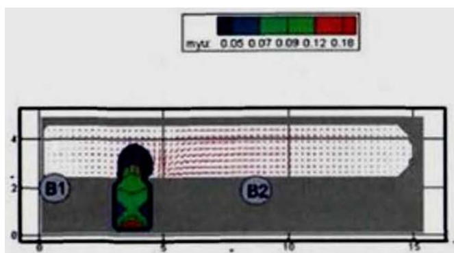
Рис. 160. Оптическая плотность дыма (Нп/м) в горизонтальном сечении на высоте 1,7 м от уровня пола в момент времени 60 с
