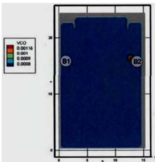
Рис. 91. Концентрация СО (кг/м 3 ) в горизонтальном сечении на высоте 2,9 м от уровня пола в момент времени 410 с
