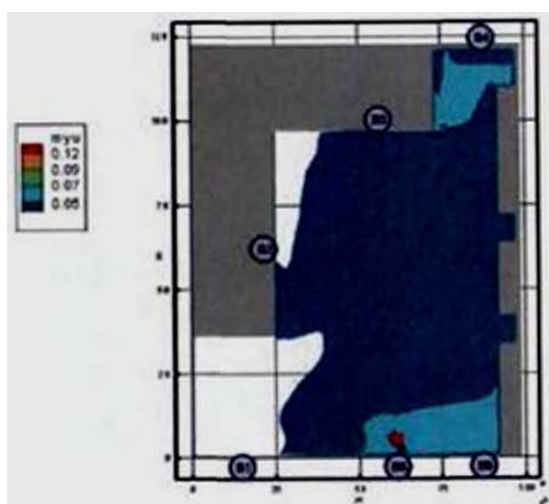
Рис. 41. Оптическая плотность дыма (Нп/м) в горизонтальном сечении на высоте 1,7 м от уровня пола в момент времени 900 с
