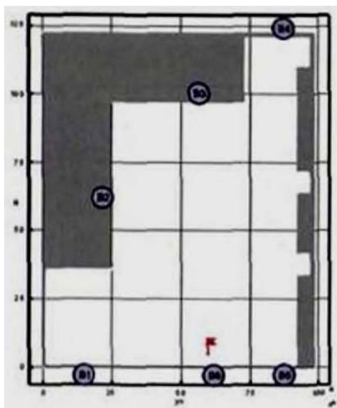
Рис. 3. Расчетная схема третьего сценария развития пожара (горизонтальное сечение на высоте 1,7 м от уровня пола): В1 - В5 эвакуационные выходы
